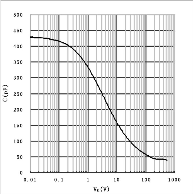
4)典型电容-反向电压曲线
